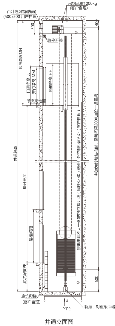
井道立面图
