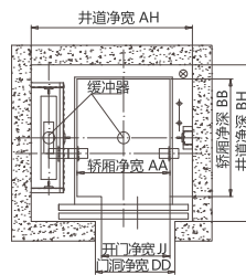
井道平面布置图
