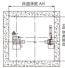
顶层井道平面布置图
