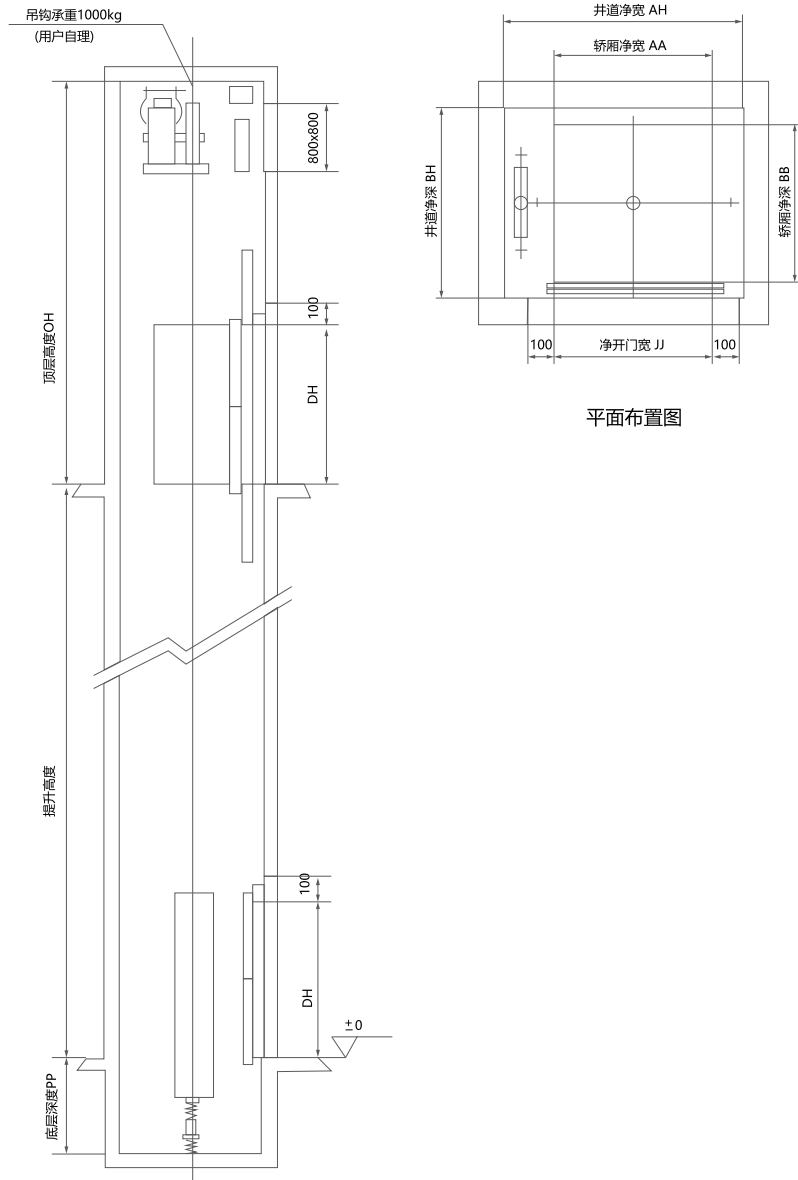
地平式立面图
